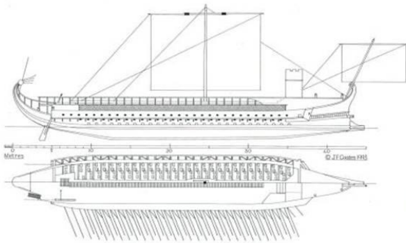
Διαγράμματα πλάγιας όψης και κάτοψης πενήτηρους σύμφωνα με τον Τζ. Φ. Κόουτς (Copyright: J.F. Coates).
